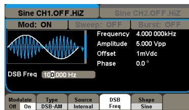
DSB-AM
