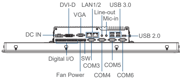
Left I/O
