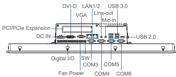
Left I/O
